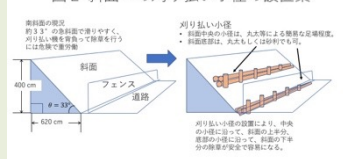
図2 斜面への刈り払い小径の設置案
